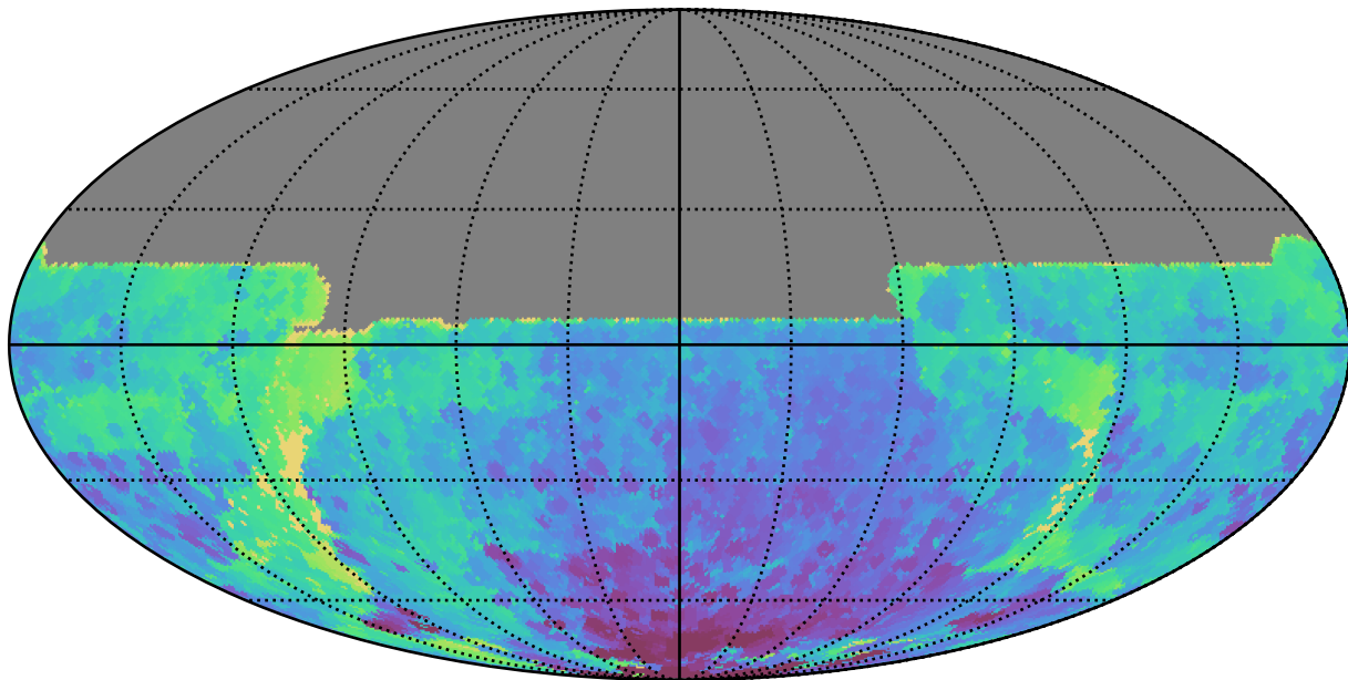
extra_ss_neo2_v3.4_10yrs All sky y band: Min HA
