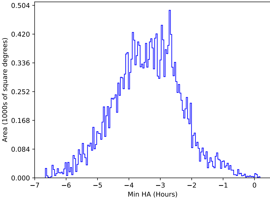
extra_ss_neo2_v3.4_10yrs All sky y band: Min HA
