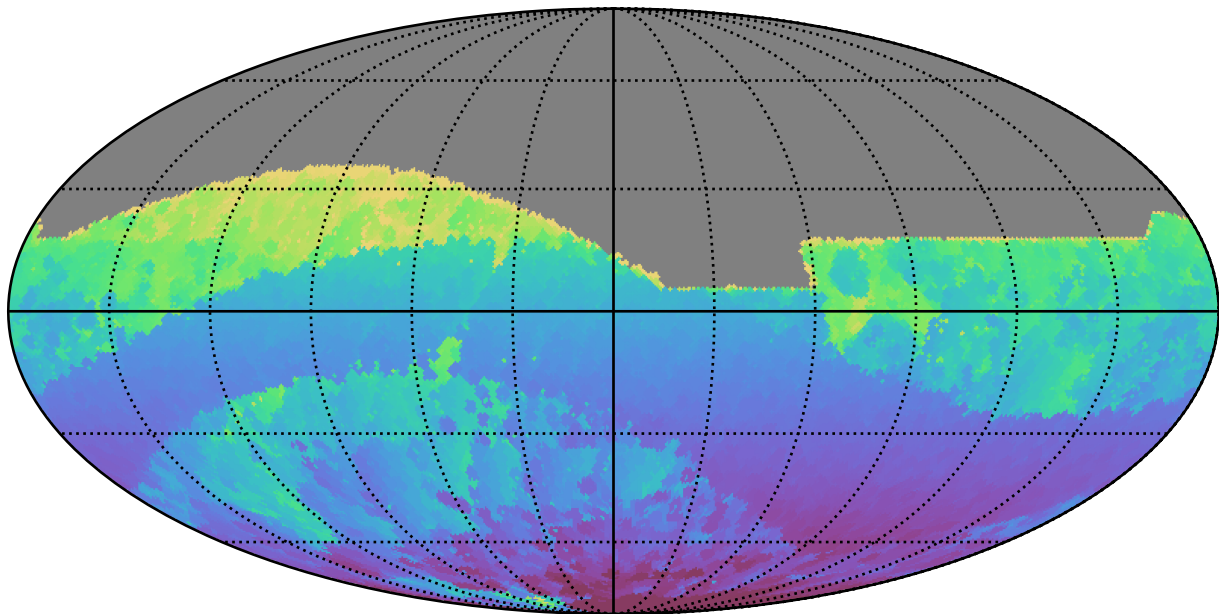
extra_ss_neo2_v3.4_10yrs All sky r band: Min HA
