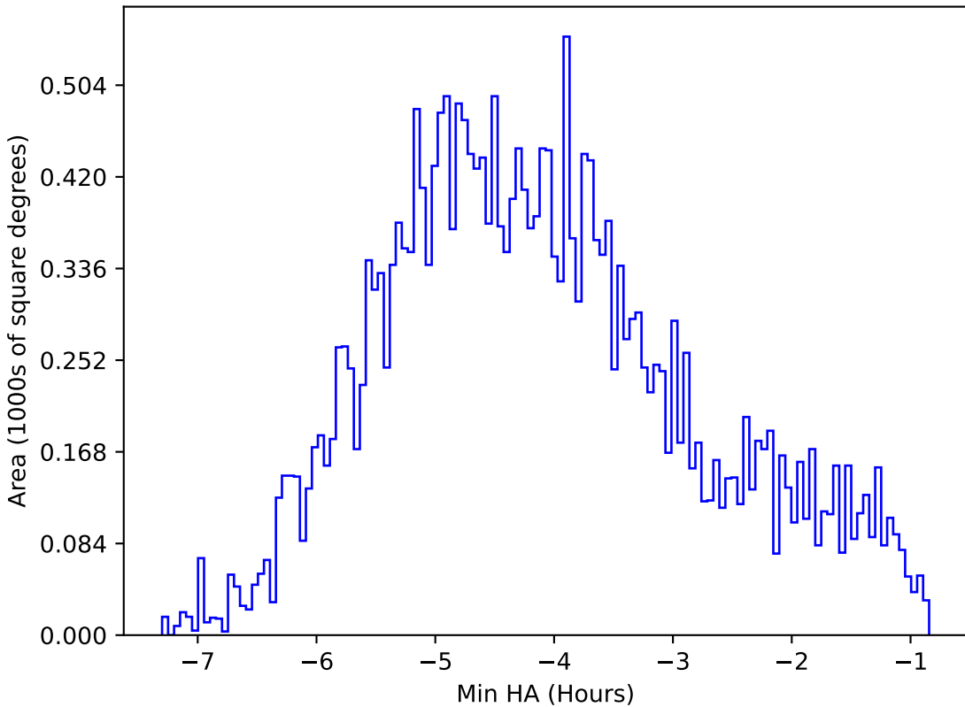
extra_ss_neo2_v3.4_10yrs All sky i band: Min HA
