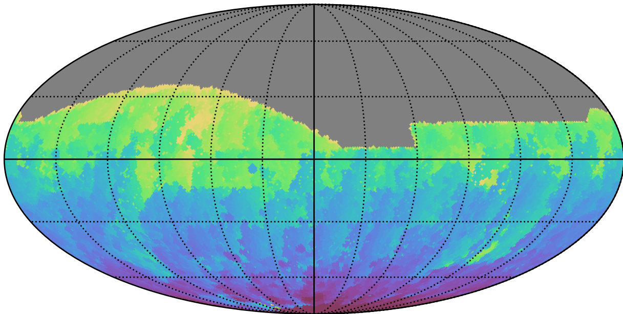
extra_ss_neo2_v3.4_10yrs All sky g band: Min HA
