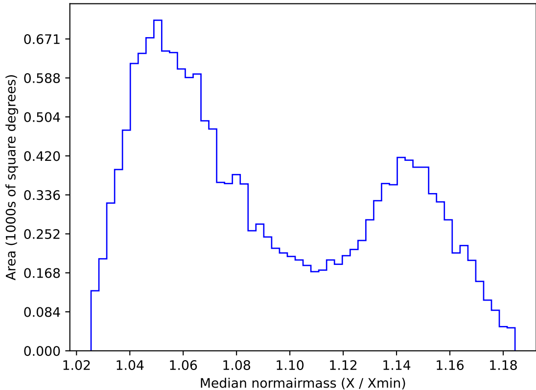
extra_ss_neo2_v3.4_10yrs WFD y band: Median normairmass
