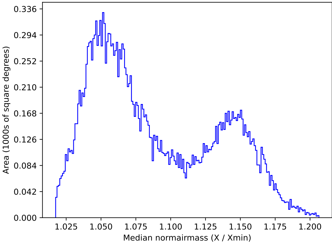
extra_ss_neo2_v3.4_10yrs All sky y band: Median normairmass
