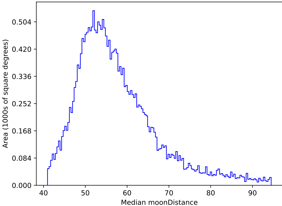
extra_ss_neo2_v3.4_10yrs All sky y band: Median moonDistance
