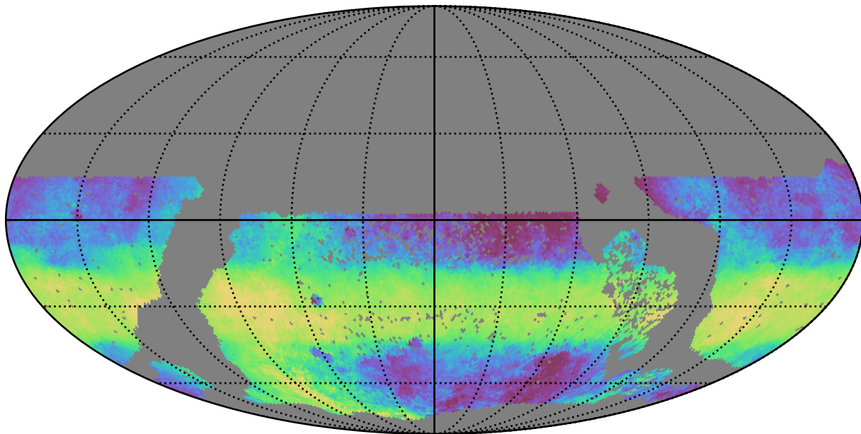
extra_ss_neo2_v3.4_10yrs WFD y band: Median HA
