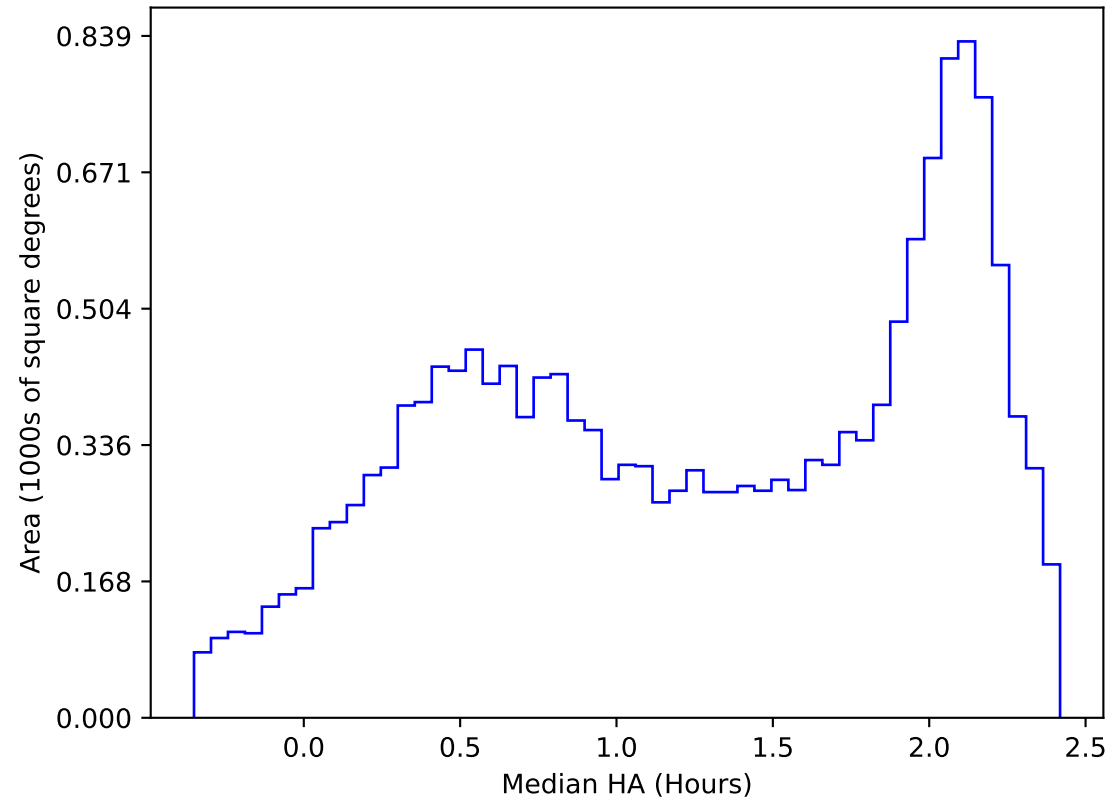
extra_ss_neo2_v3.4_10yrs WFD y band: Median HA
