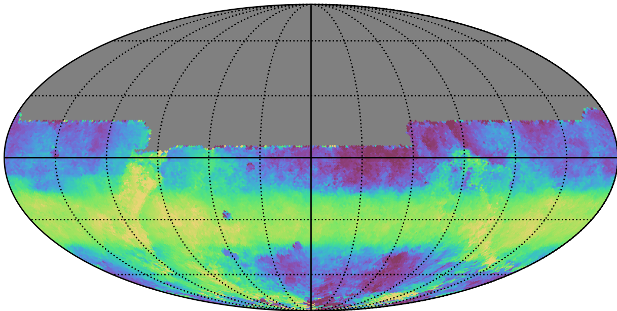
extra_ss_neo2_v3.4_10yrs All sky y band: Median HA
