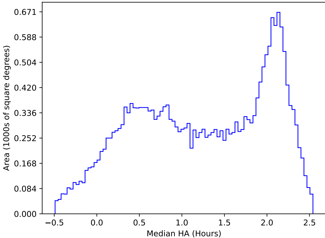
extra_ss_neo2_v3.4_10yrs All sky y band: Median HA
