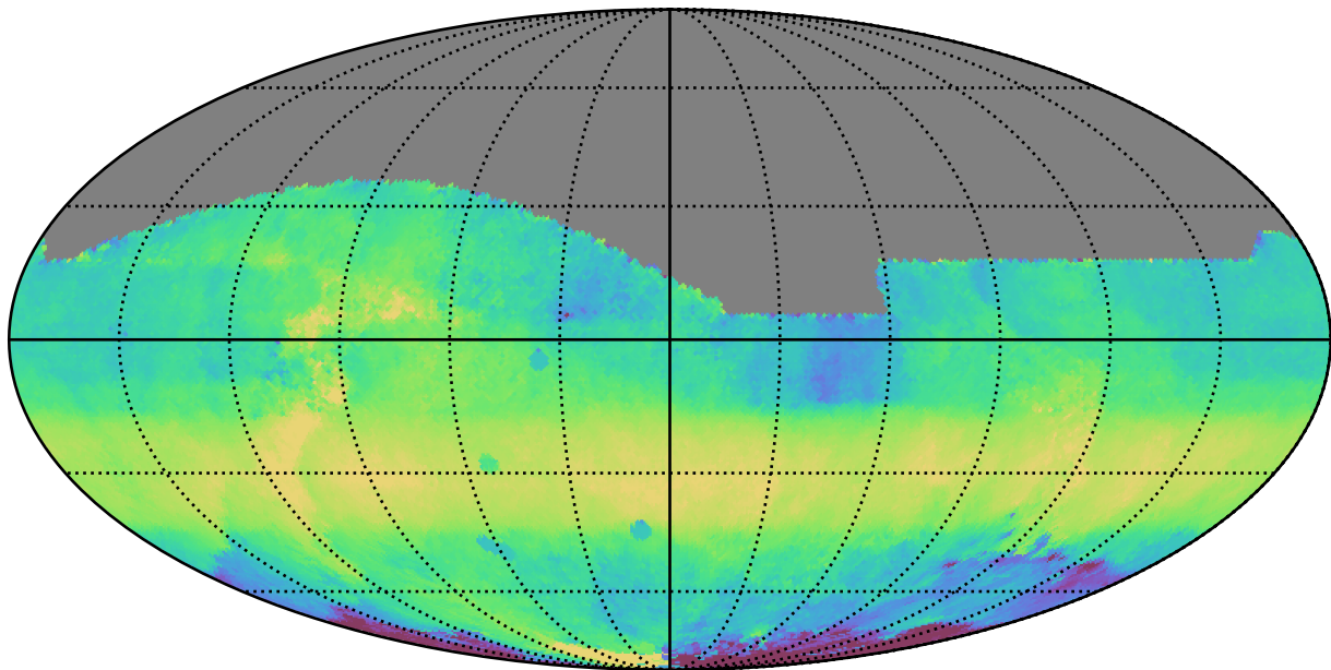
extra_ss_neo2_v3.4_10yrs All sky i band: Median HA
