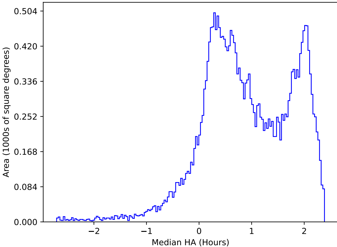
extra_ss_neo2_v3.4_10yrs All sky i band: Median HA
