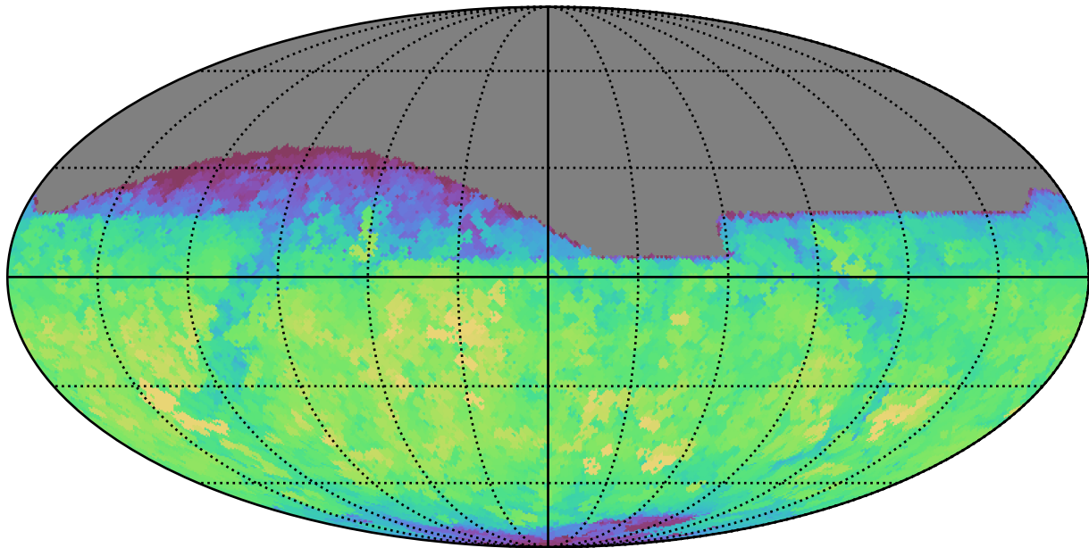
extra_ss_neo2_v3.4_10yrs All sky z band: Max saturation_mag
