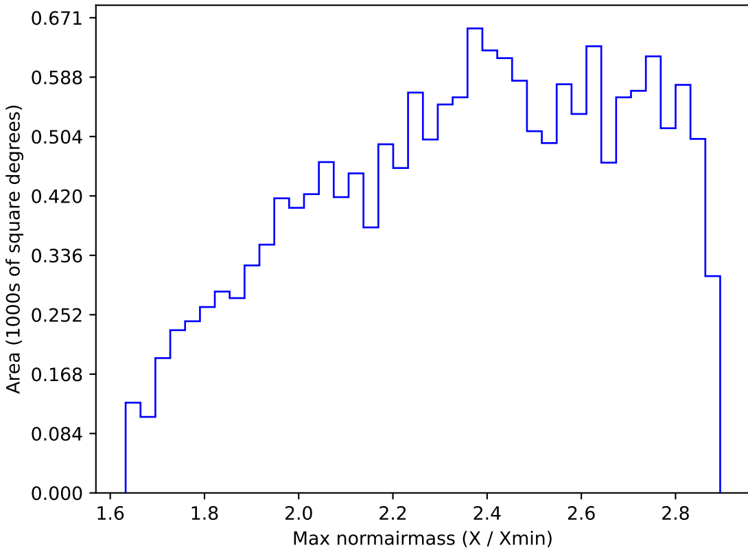
extra_ss_neo2_v3.4_10yrs WFD z band: Max normairmass
