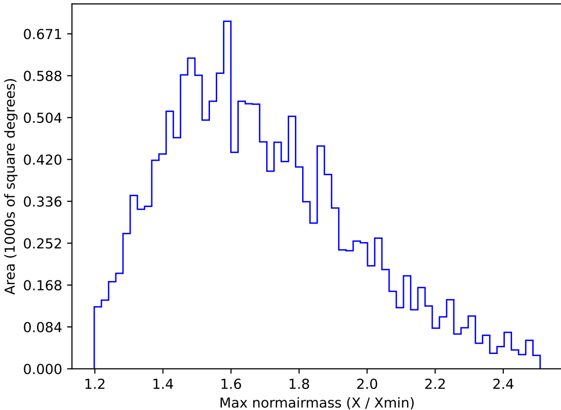
extra_ss_neo2_v3.4_10yrs WFD u band: Max normairmass
