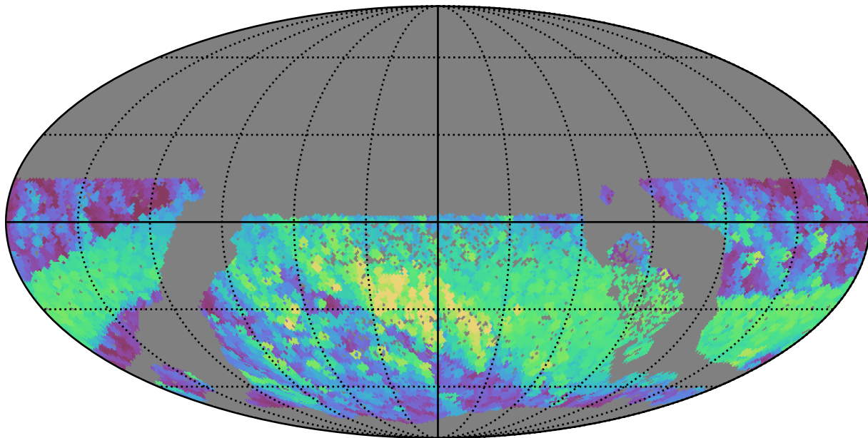
extra_ss_neo2_v3.4_10yrs WFD r band: Max normairmass
