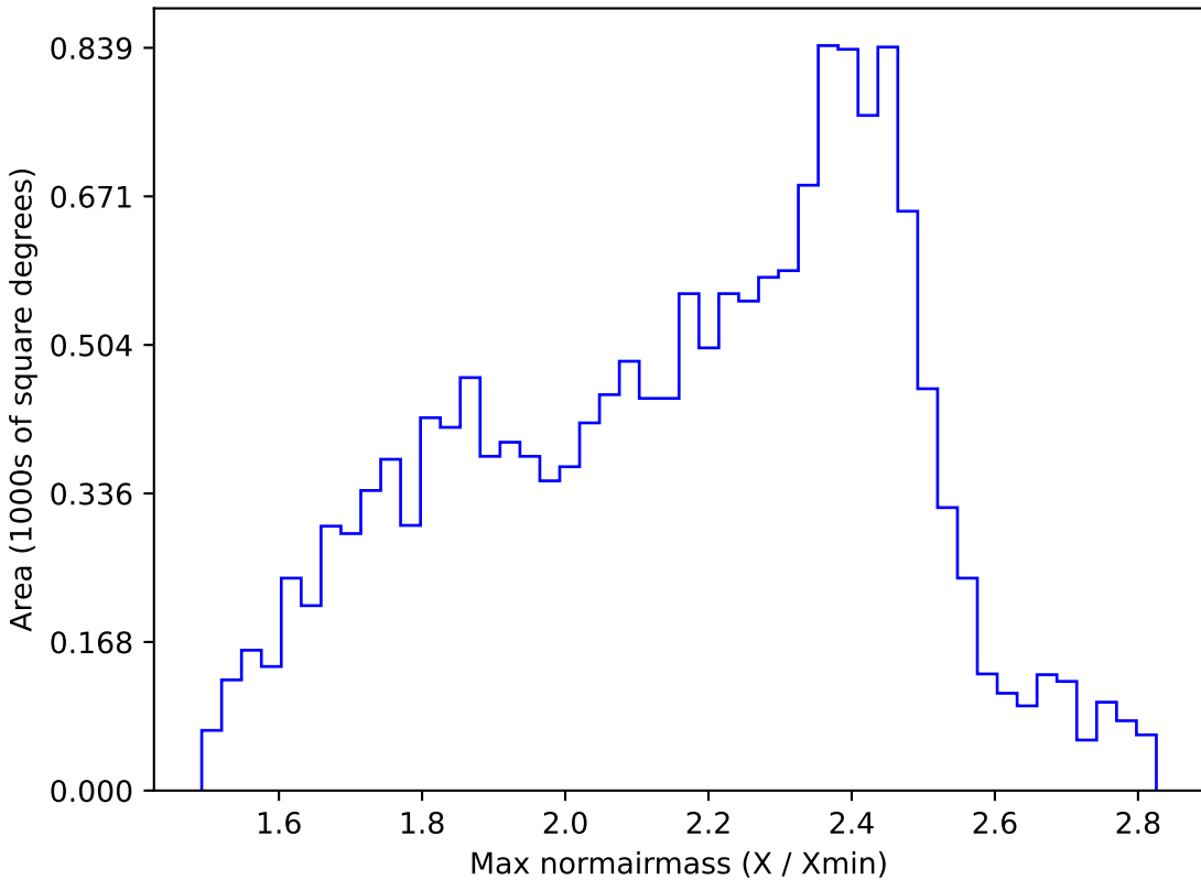
extra_ss_neo2_v3.4_10yrs WFD r band: Max normairmass
