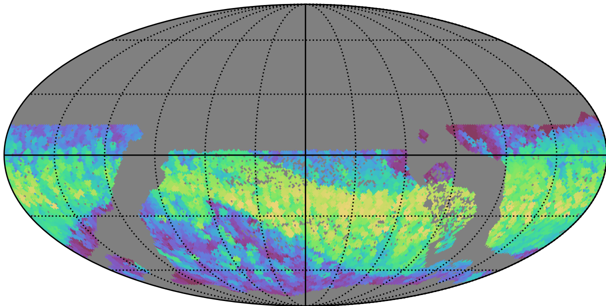
extra_ss_neo2_v3.4_10yrs WFD i band: Max normairmass
