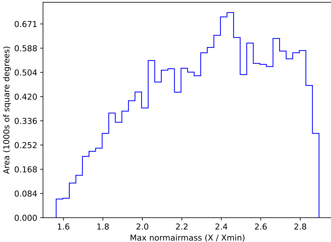
extra_ss_neo2_v3.4_10yrs WFD i band: Max normairmass
