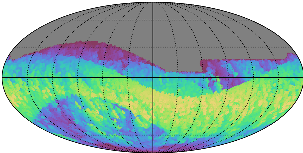
extra_ss_neo2_v3.4_10yrs All sky z band: Max normairmass
