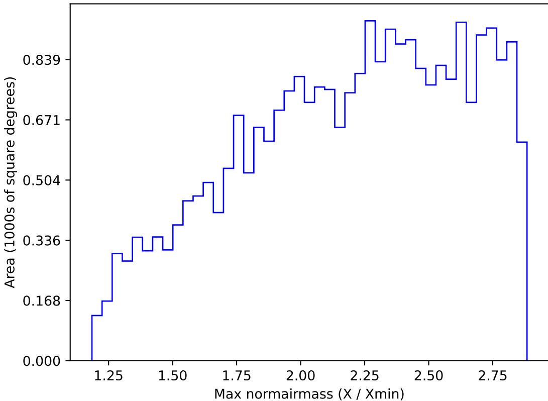
extra_ss_neo2_v3.4_10yrs All sky z band: Max normairmass
