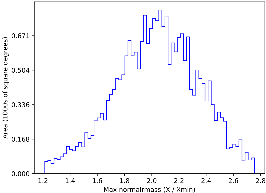
extra_ss_neo2_v3.4_10yrs All sky y band: Max normairmass
