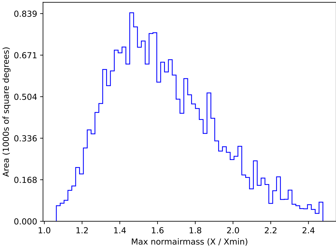
extra_ss_neo2_v3.4_10yrs All sky u band: Max normairmass
