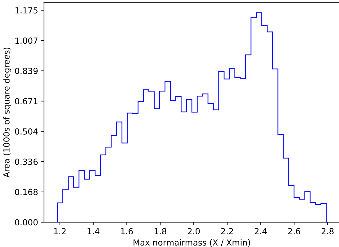
extra_ss_neo2_v3.4_10yrs All sky r band: Max normairmass
