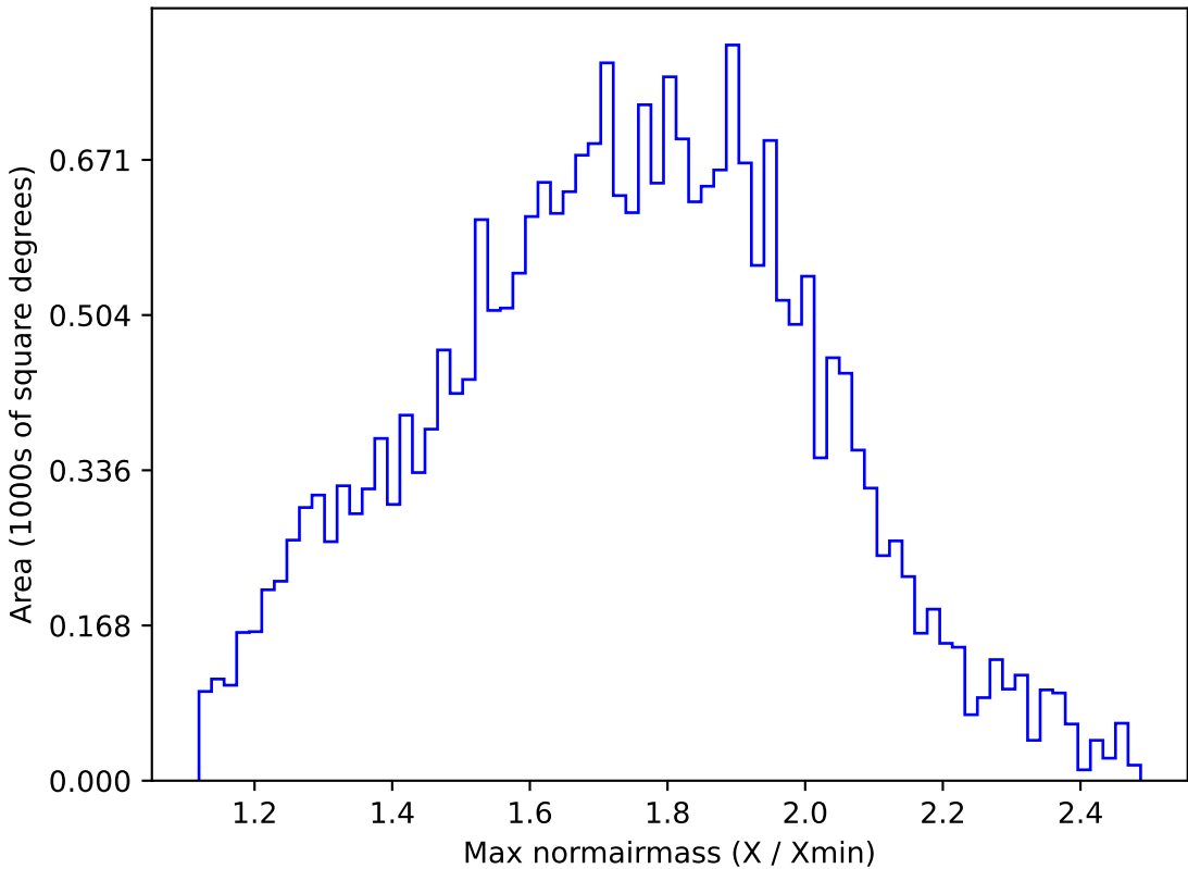
extra_ss_neo2_v3.4_10yrs All sky g band: Max normairmass
