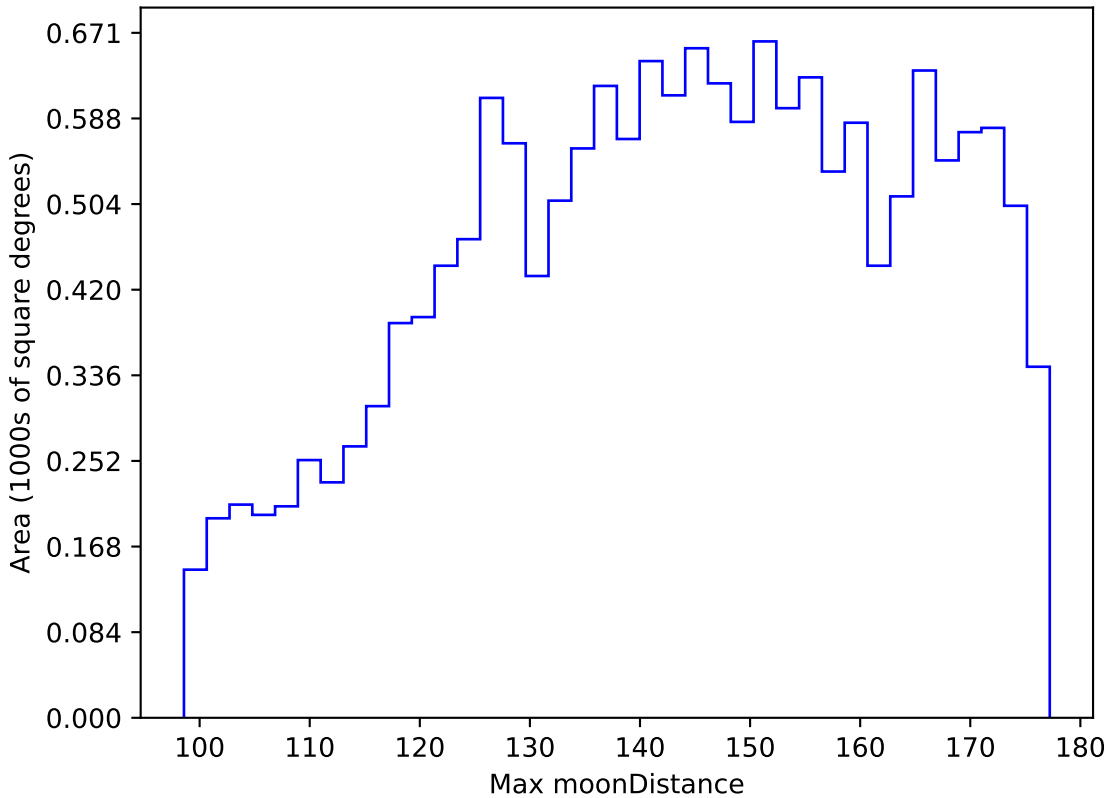
extra_ss_neo2_v3.4_10yrs WFD y band: Max moonDistance
