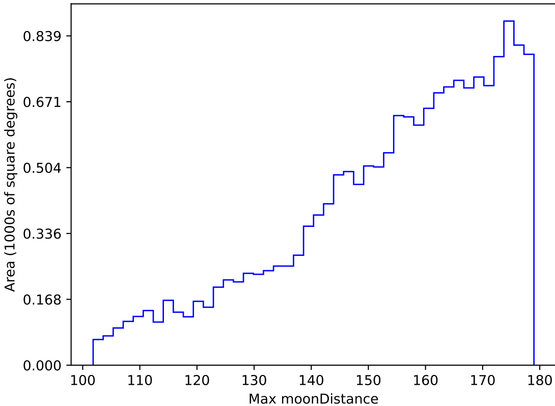
extra_ss_neo2_v3.4_10yrs WFD u band: Max moonDistance
