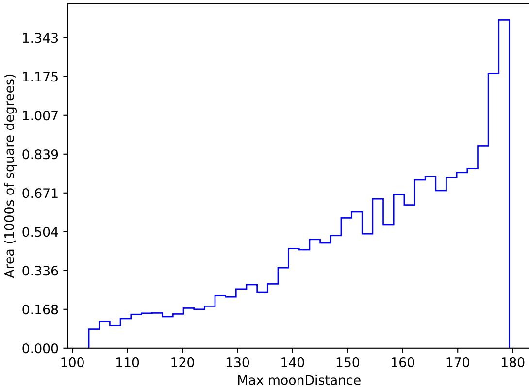
extra_ss_neo2_v3.4_10yrs WFD r band: Max moonDistance
