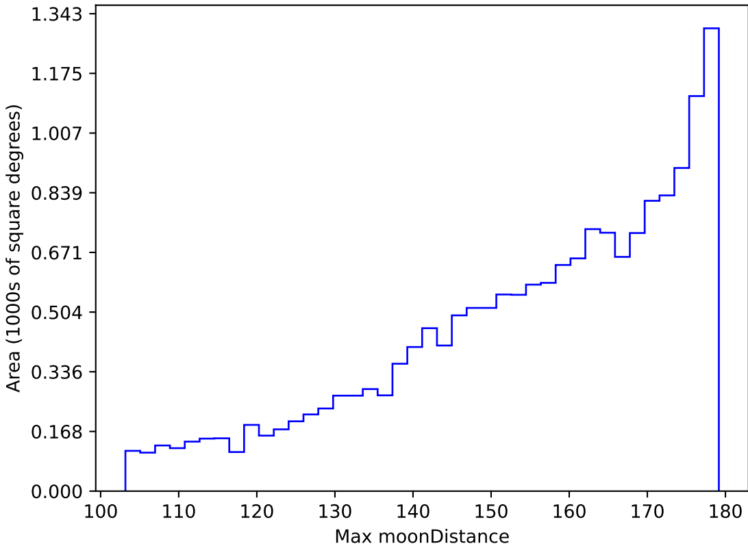
extra_ss_neo2_v3.4_10yrs WFD i band: Max moonDistance
