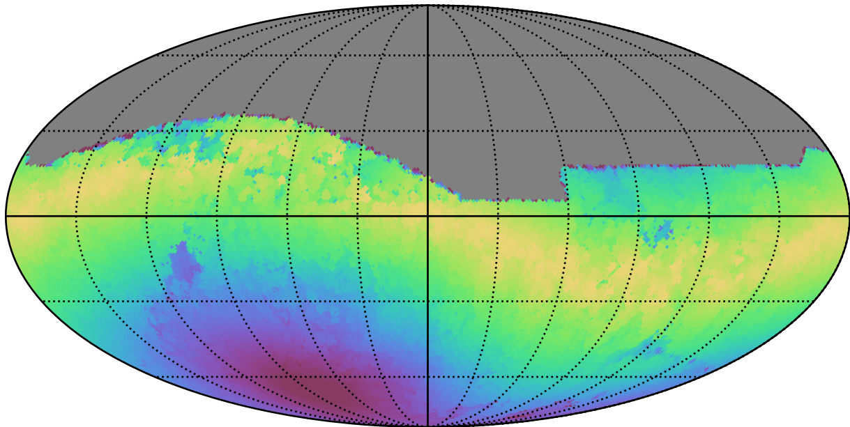
extra_ss_neo2_v3.4_10yrs All sky z band: Max moonDistance
