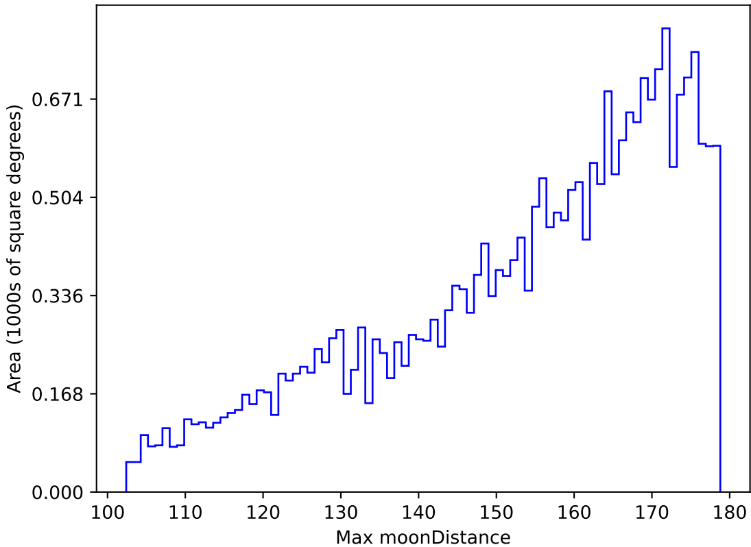
extra_ss_neo2_v3.4_10yrs All sky z band: Max moonDistance
