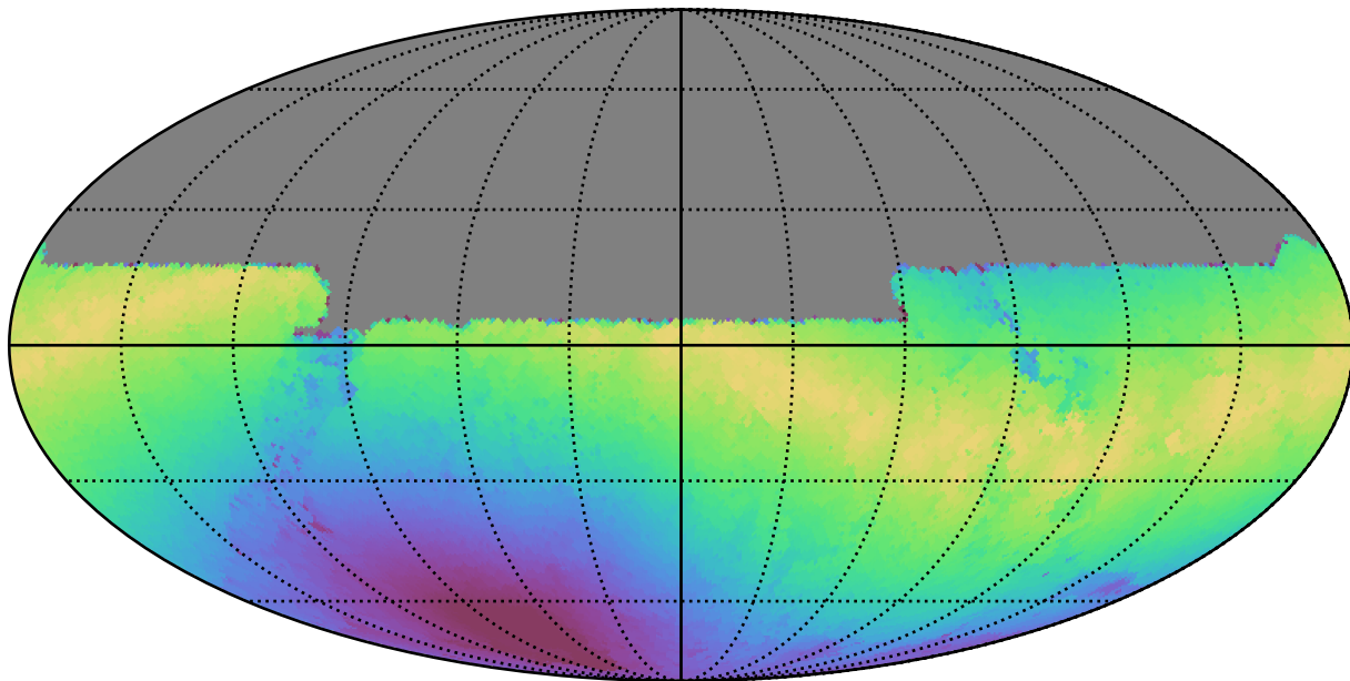
extra_ss_neo2_v3.4_10yrs All sky u band: Max moonDistance
