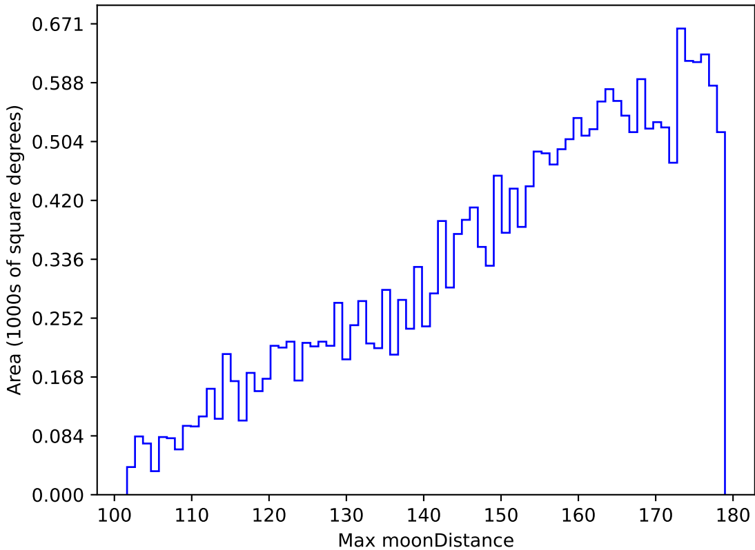
extra_ss_neo2_v3.4_10yrs All sky u band: Max moonDistance
