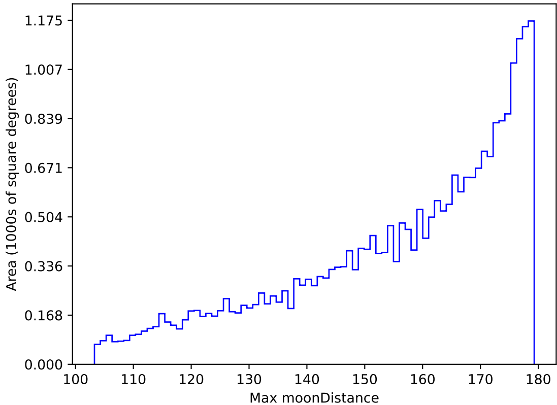
extra_ss_neo2_v3.4_10yrs All sky r band: Max moonDistance
