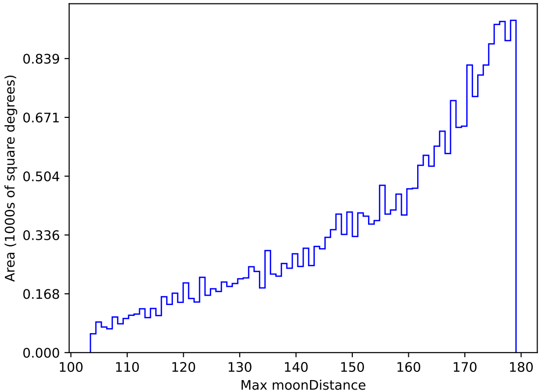
extra_ss_neo2_v3.4_10yrs All sky i band: Max moonDistance
