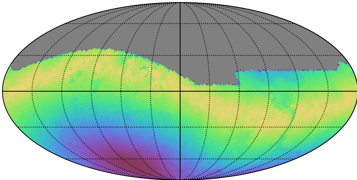
extra_ss_neo2_v3.4_10yrs All sky g band: Max moonDistance
