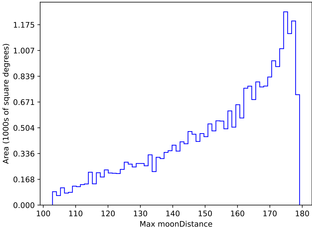
extra_ss_neo2_v3.4_10yrs All sky g band: Max moonDistance
