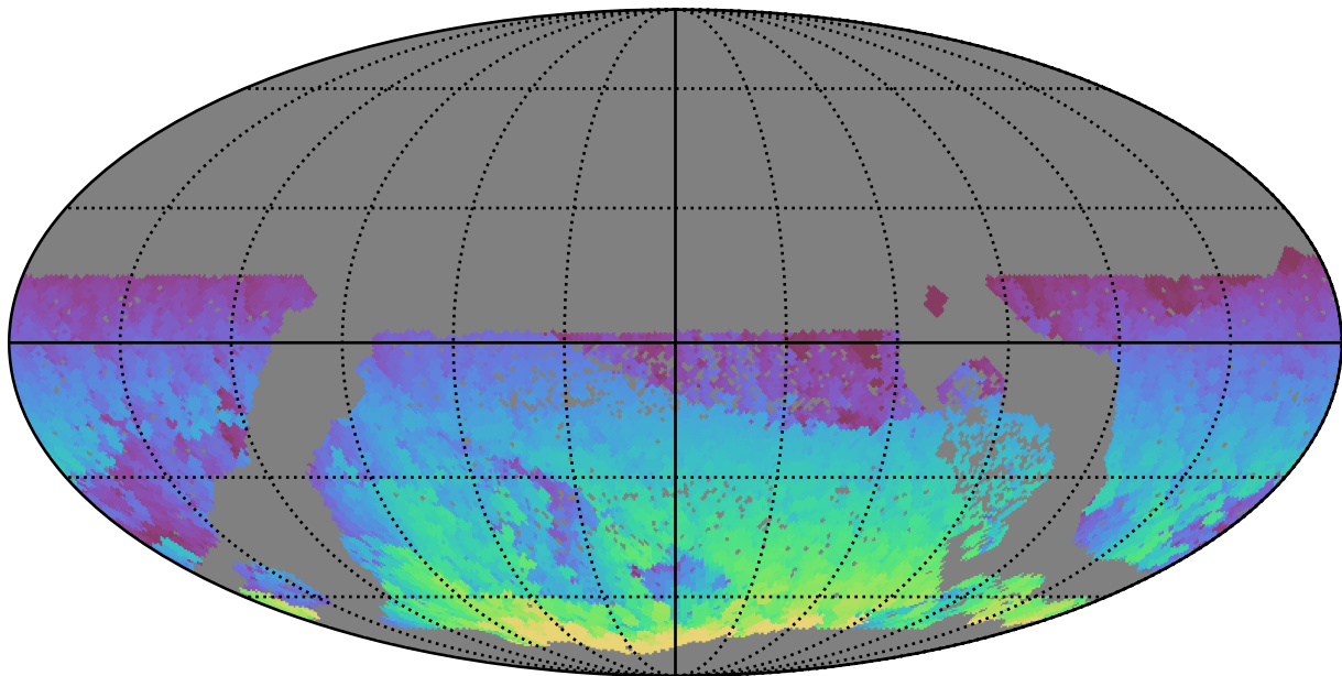
extra_ss_neo2_v3.4_10yrs WFD z band: Max HA
