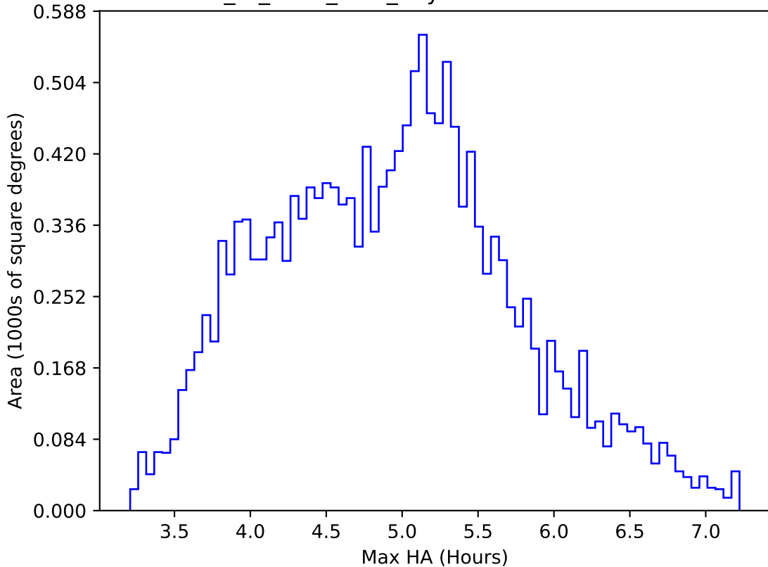
extra_ss_neo2_v3.4_10yrs WFD z band: Max HA
