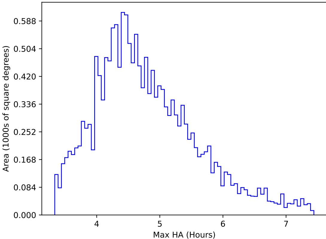
extra_ss_neo2_v3.4_10yrs WFD y band: Max HA
