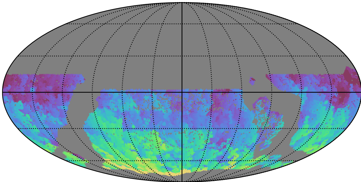
extra_ss_neo2_v3.4_10yrs WFD u band: Max HA
