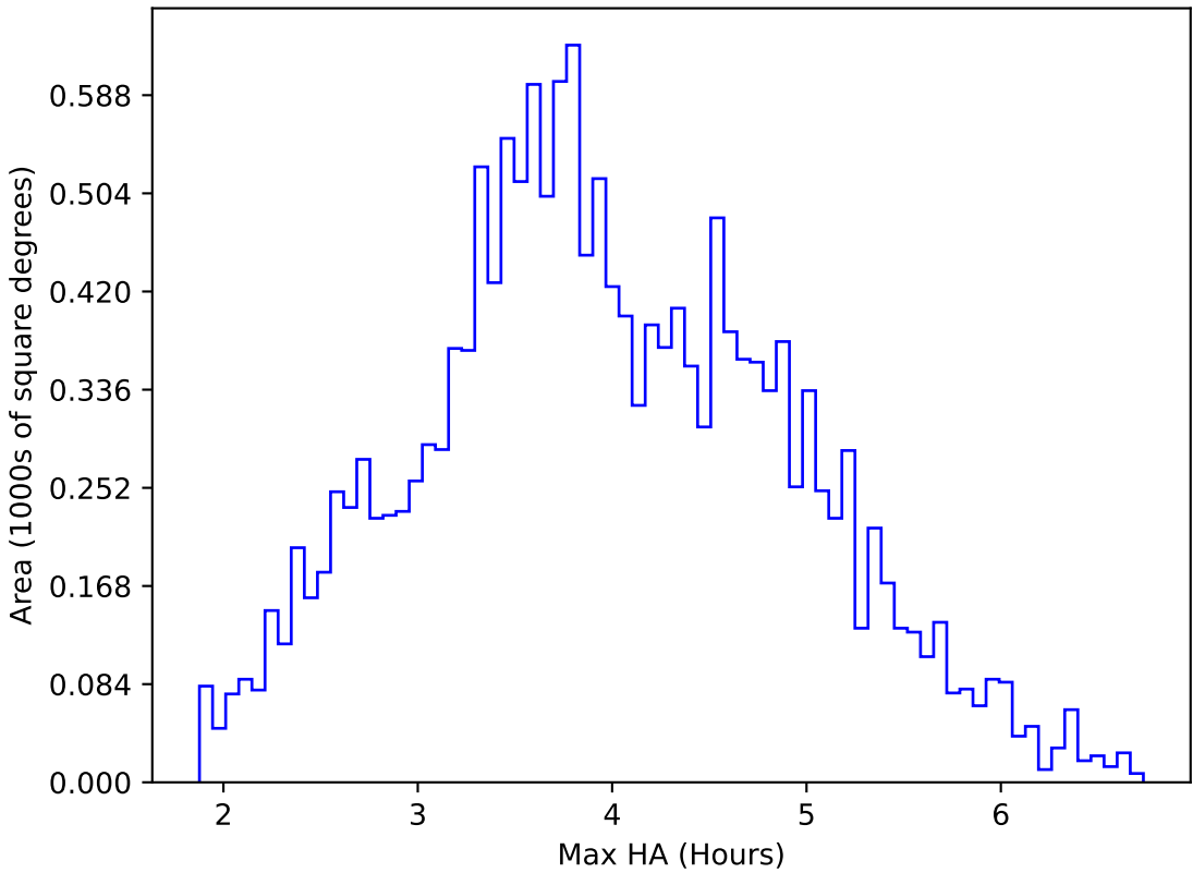
extra_ss_neo2_v3.4_10yrs WFD u band: Max HA
