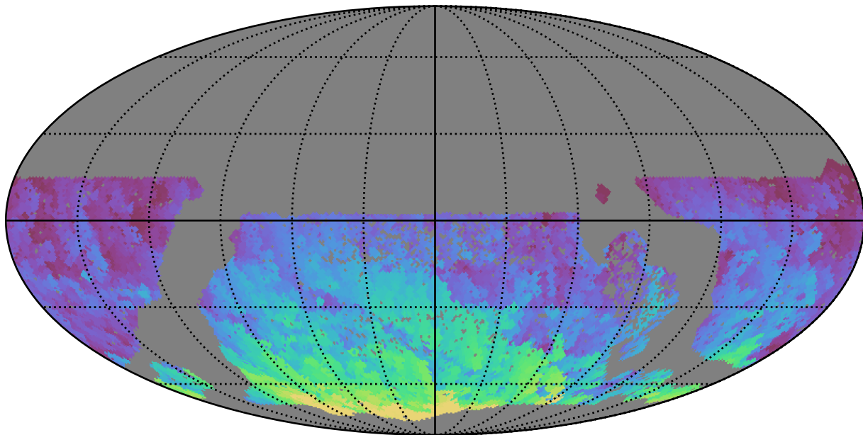
extra_ss_neo2_v3.4_10yrs WFD r band: Max HA
