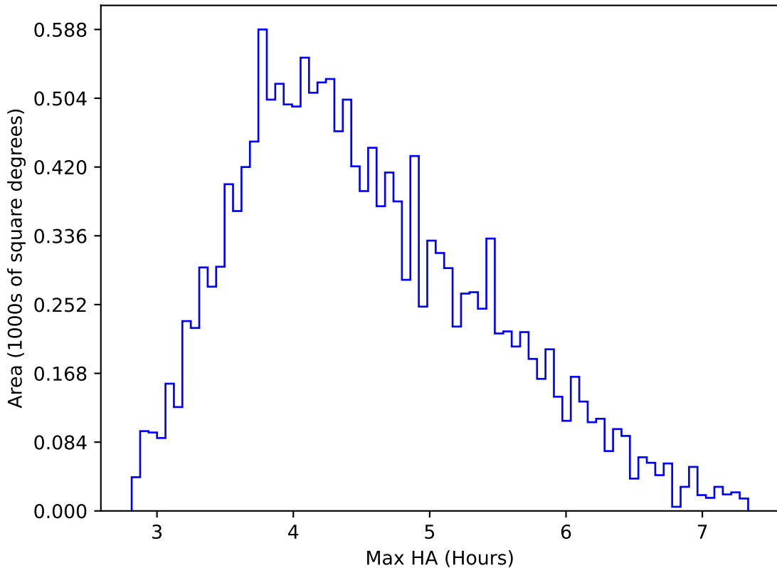
extra_ss_neo2_v3.4_10yrs WFD r band: Max HA
