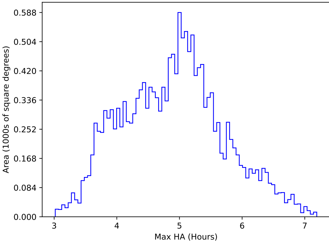
extra_ss_neo2_v3.4_10yrs WFD i band: Max HA
