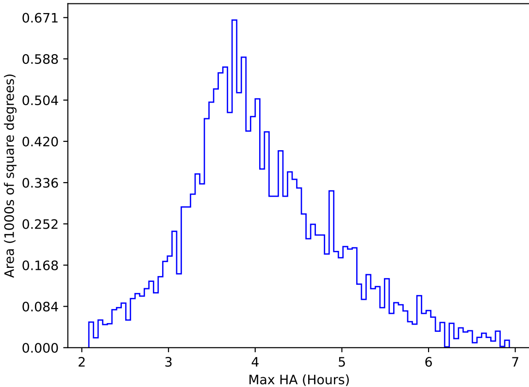
extra_ss_neo2_v3.4_10yrs WFD g band: Max HA
