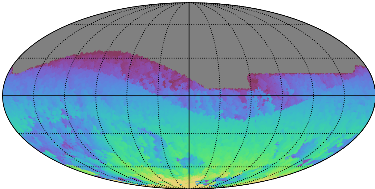
extra_ss_neo2_v3.4_10yrs All sky z band: Max HA
