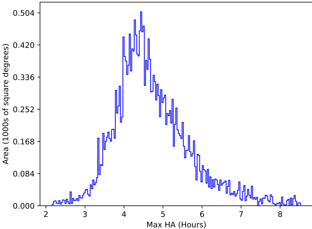
extra_ss_neo2_v3.4_10yrs All sky y band: Max HA
